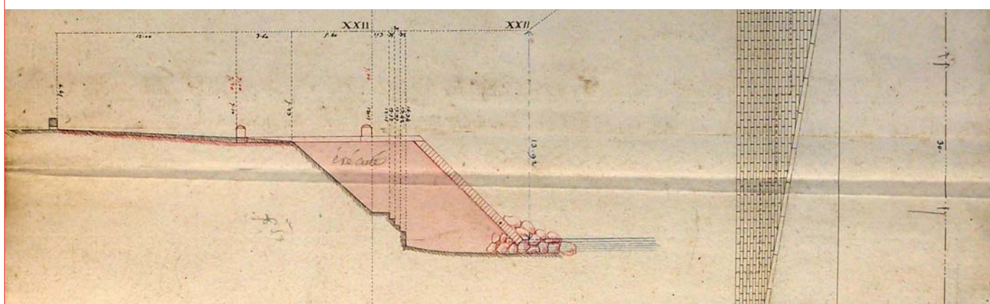
Profils en travers du nouveau quai Saint-Clair n°XXII (en bas) et XXIII (en haut), 1823
